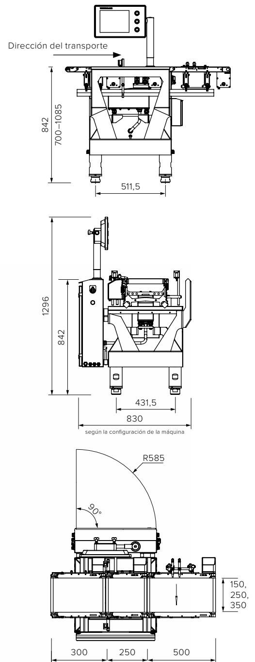
Todos los datos en mm | La imagen muestra un modelo de ejemplo
