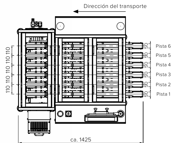
Todos los datos en mm | La imagen muestra un modelo de ejemplo
