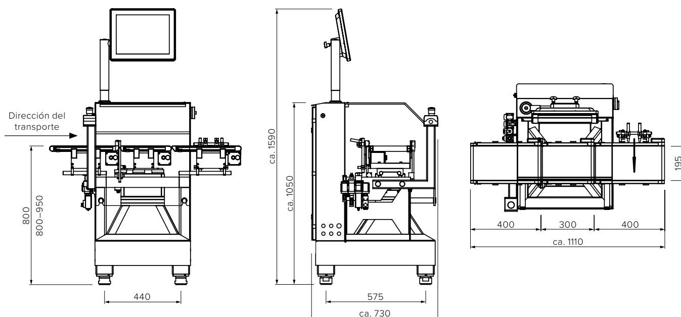
Refinada técnica de pesaje HC-A también como variante multipista
